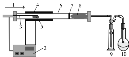
1—载气(氮气/空气); 2—温控装置; 3—热电偶; 4—加热套管; 5—石英舟; 6—石英管; 7—石英棉; 8—XAD-2树脂; 9—气体 收集瓶; 10—气体收集瓶(甲苯溶液)。
